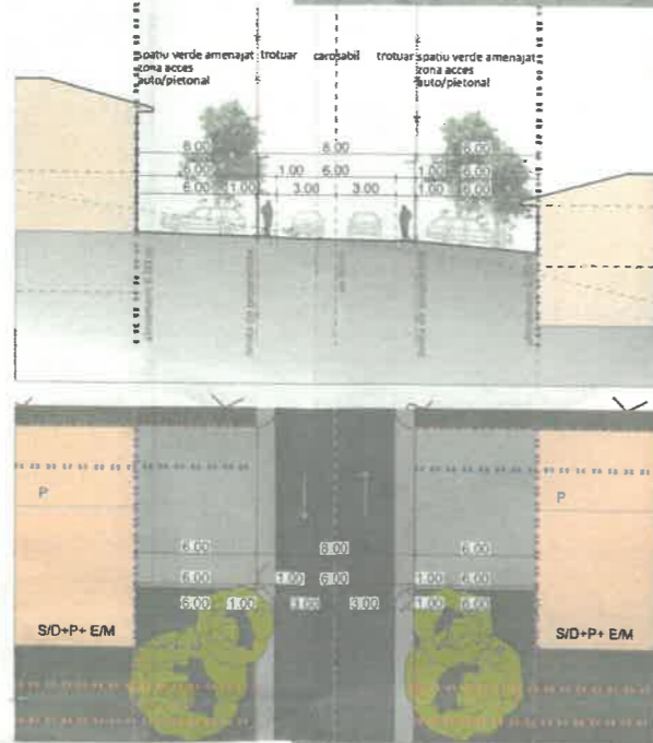
PROFIL STRADAL 1-1
